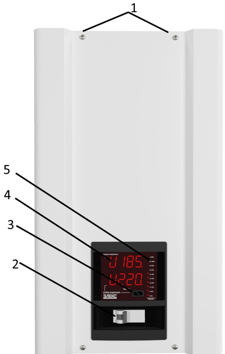
Рис.1 Внешний вид стабилизатора
