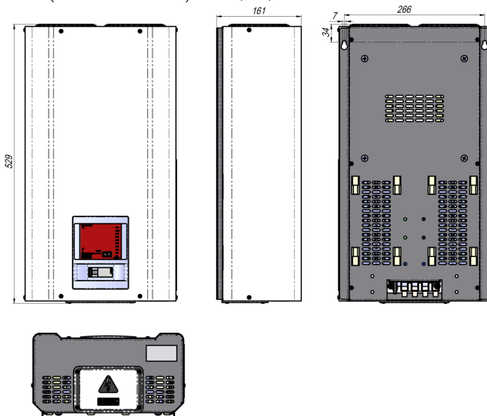
Рисунок 5. Габаритные и установочные размеры стабилизаторов АМПЕР (9/12/16 точный) на 50, 63 и 80А и АМПЕР-Р на 40, 50, 63, 80А
