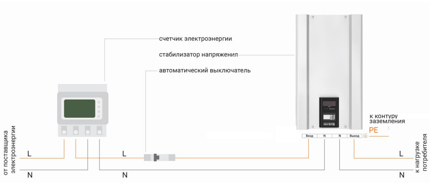
Рисунок 6. Схема подключения стабилизатора к однофазной сети
