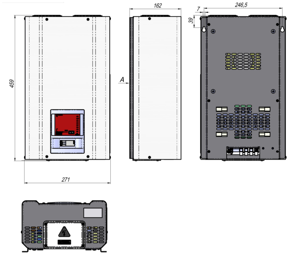
Рисунок 4. Габаритные и установочные размеры стабилизаторов АМПЕР (9/12/16 точный) на 25, 32, 40А и АМПЕР-Р на 25 и 32А.
