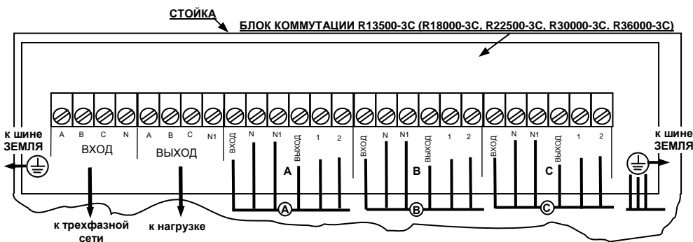
а) подключение блока коммутации
