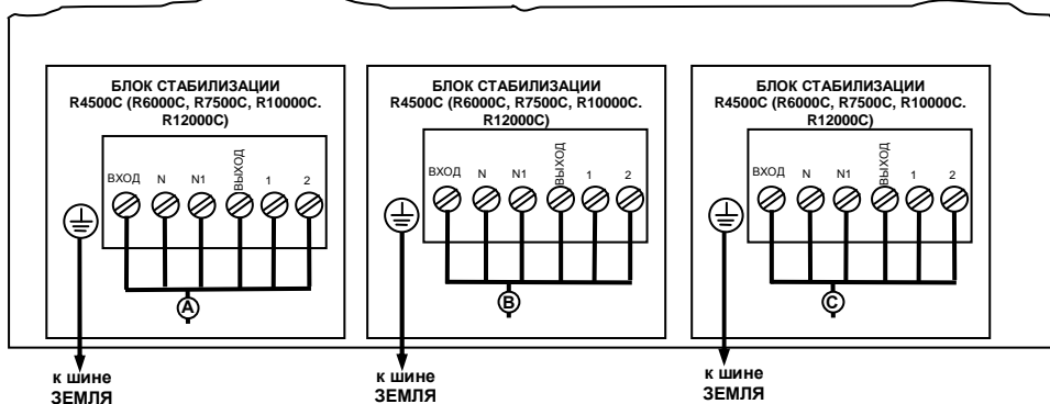
б) подключение блоков стабилизации
