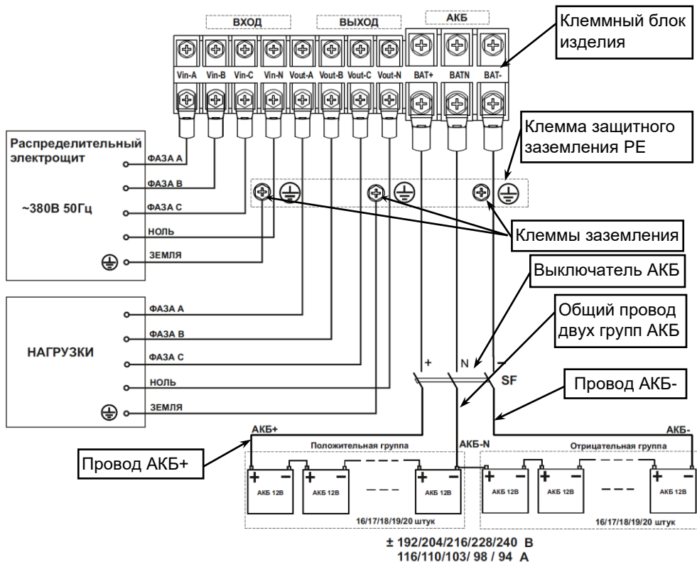
Рисунок 23 — Схема подключения изделия и монтажа аккумуляторной батареи.
